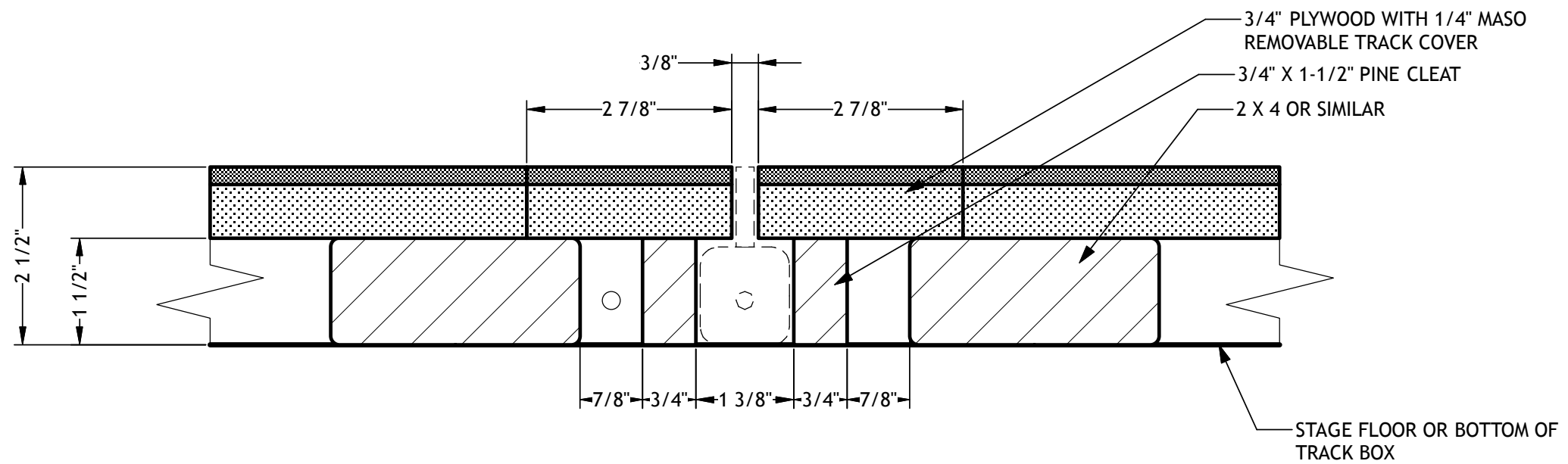
SECTION - TRACK BOX scale: 1:1
